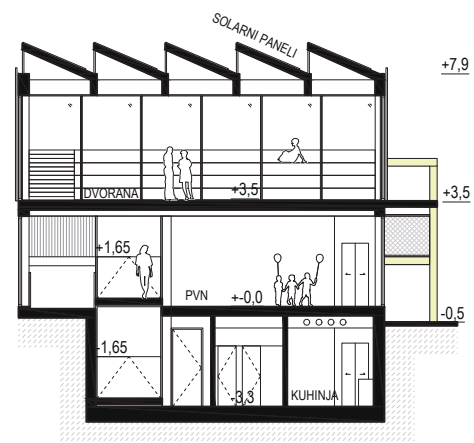
PRESJEK 2-2
