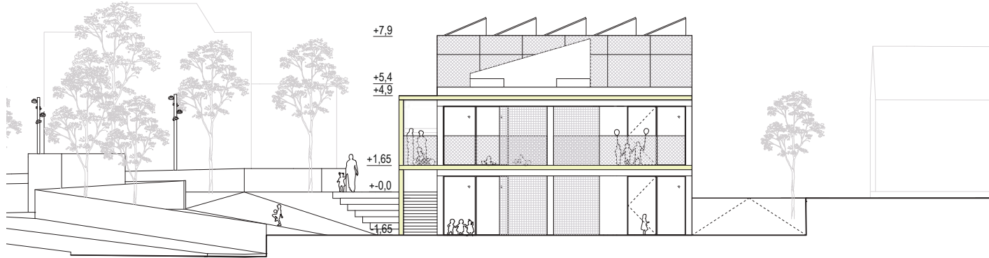
ISTOČNA FASADA
