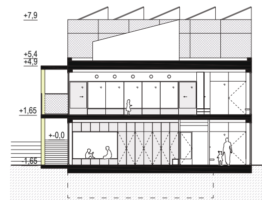
PRESJEK 3-3
