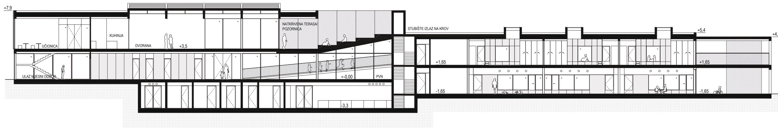
PRESJEK 1-1
