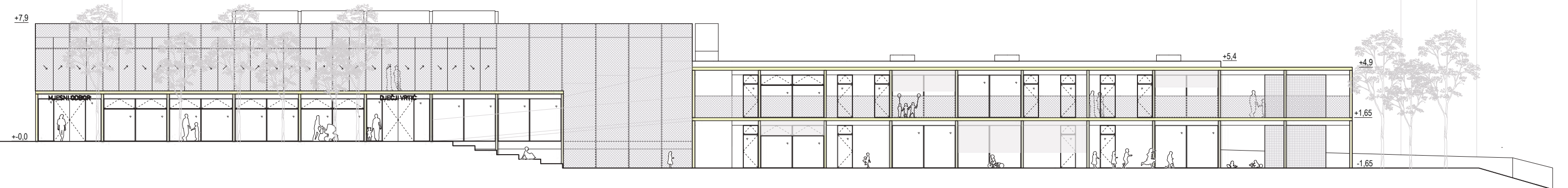
JUŽNA FASADA
